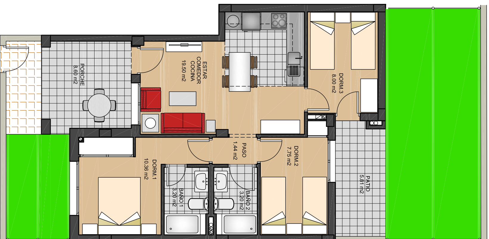
PLANTA BAJA
